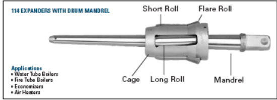
EXPANSOR DE TUBOS CON CAMPANA
