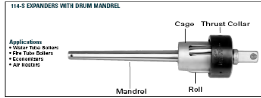
EXPANSOR DE TUBOS RECTO
